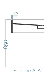
Sezione A-A'
